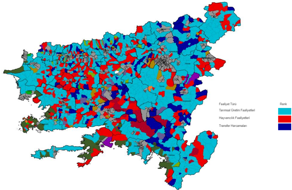
Şekil 17.Ana Geçim Kaynakları
