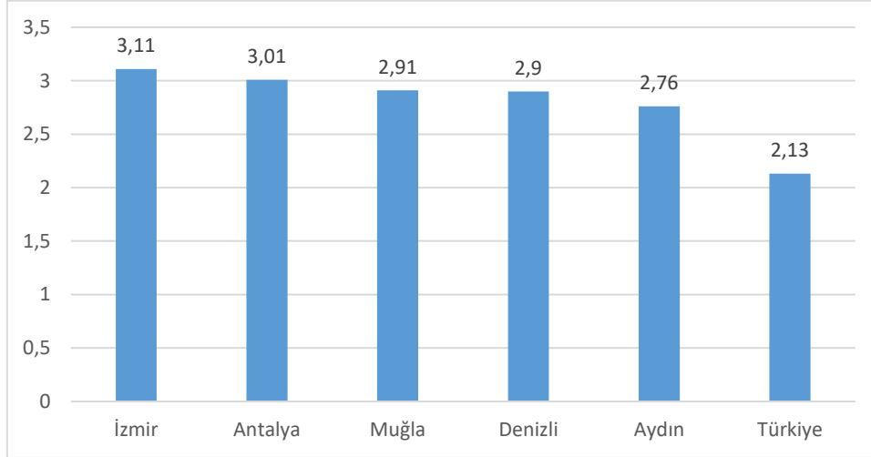
Şekil 12.Kaba Boşanma Hızı (%)
