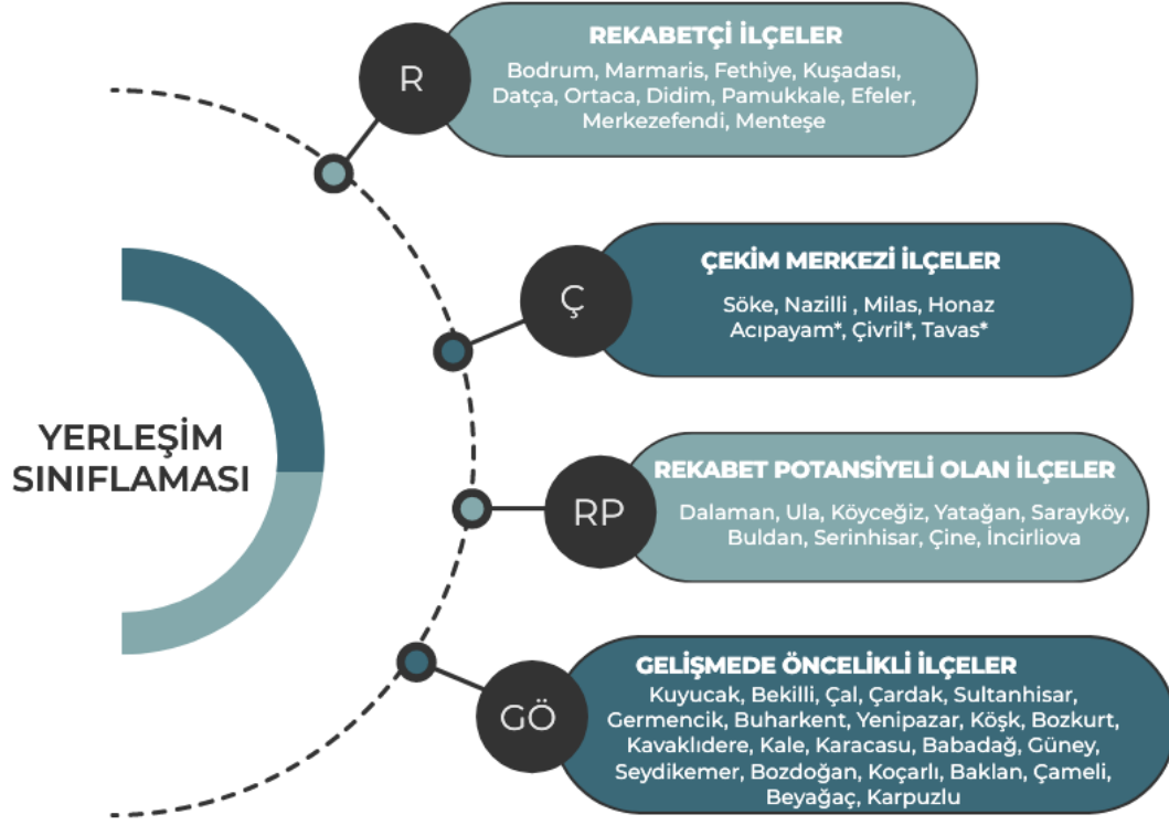
Şekil 5.Yerleşim Sınıflaması
