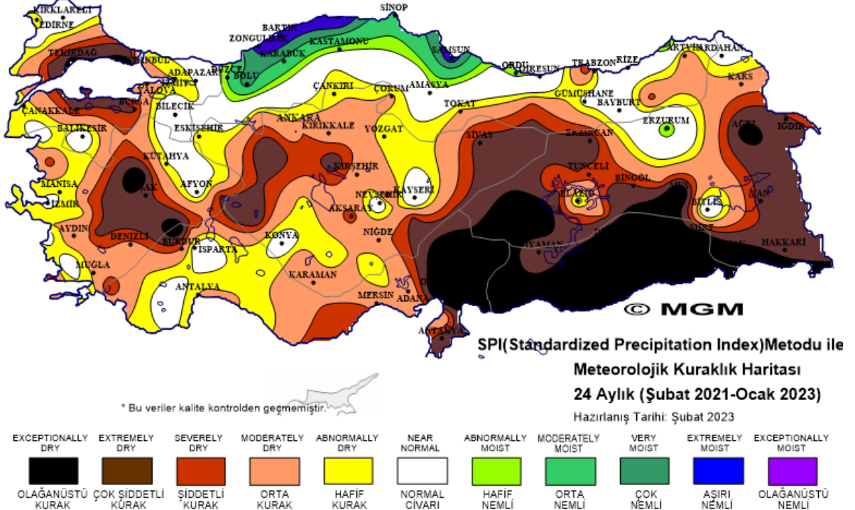
Şekil 15. Kuraklık Haritası
