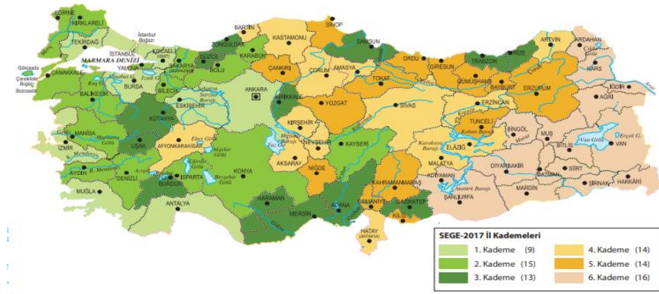
Şekil 3.İllerin Gelişmişlik Kademeleri
